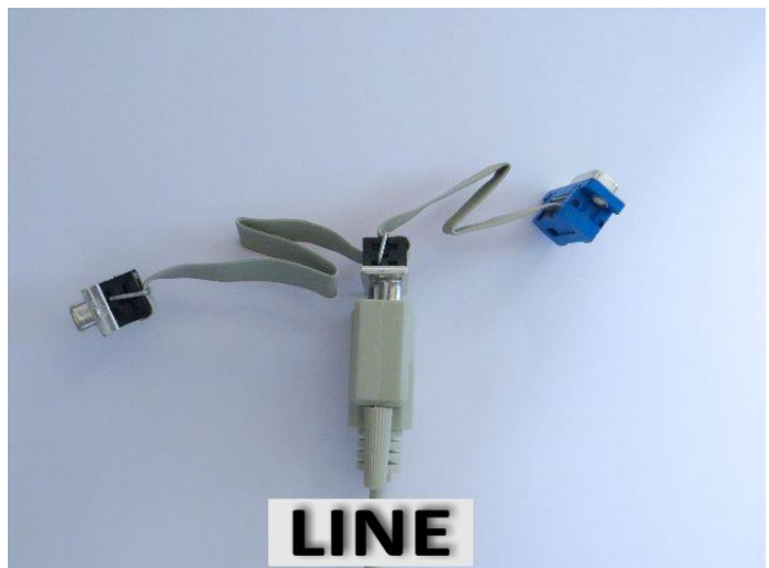
Abb.7.f: Anschluss LINE-Leitung an TESTLINE-Kabel
