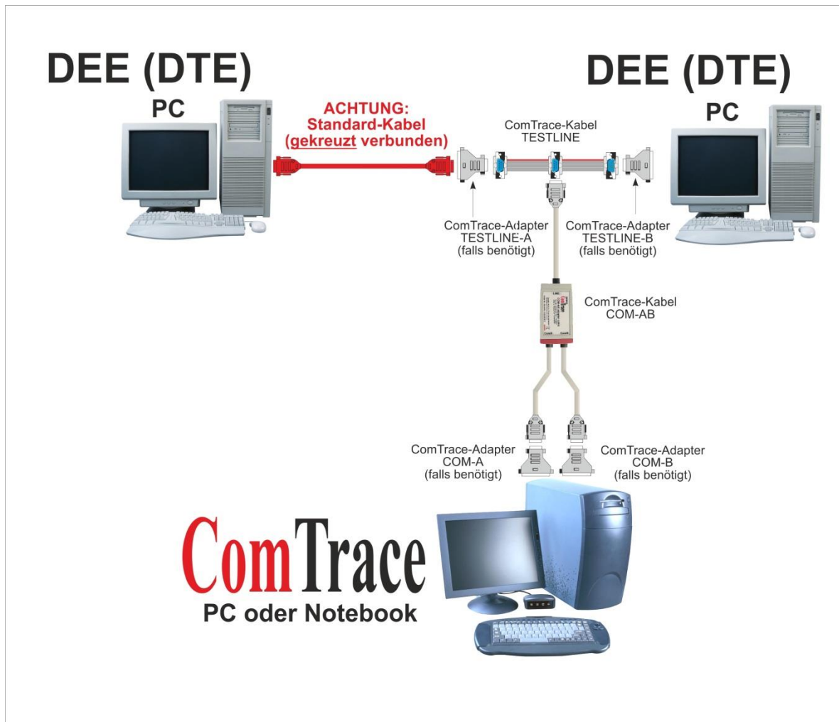
Abb.9.c: Messaufbau (Beispiel 2-B) – DEE/DEE-Verbindung (z.B. PC-PC)
